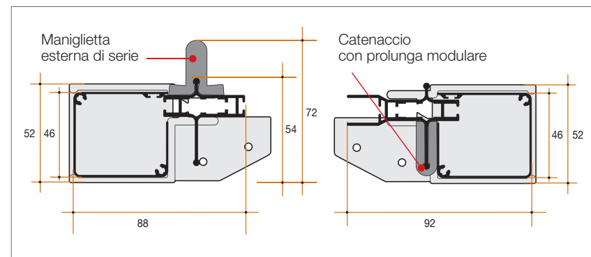
Ingombri versione a due battenti
