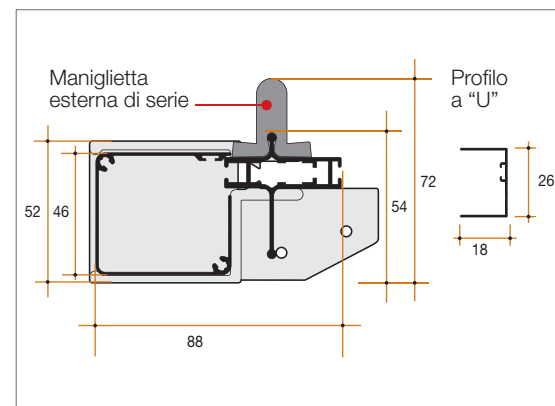
Ingombri versione a due battenti
